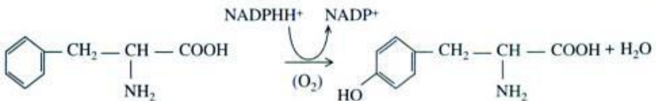
Phénylalanine
